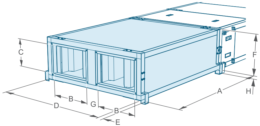
EVCBVA---/ DS (double skinned 25mm)
